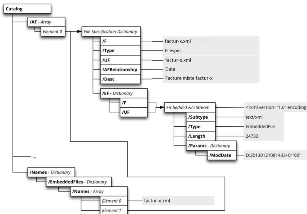
Structure du PDF/A-3 pour le fichier embarqué en XML Factur-X
